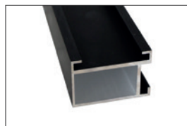
Aufbauhöhe 40 mm für die sichtbare Befestigung von Holz- oder WPC-Dielen. Tragweite 95 cm.
