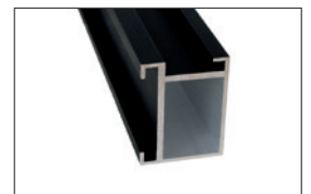
Aufbauhöhe 60 mm mit erhöhter Tragweite für die sichtbare bzw. unsichtbare Befestigung von Holz- oder WPC-Dielen. Tragweite 130 cm.
